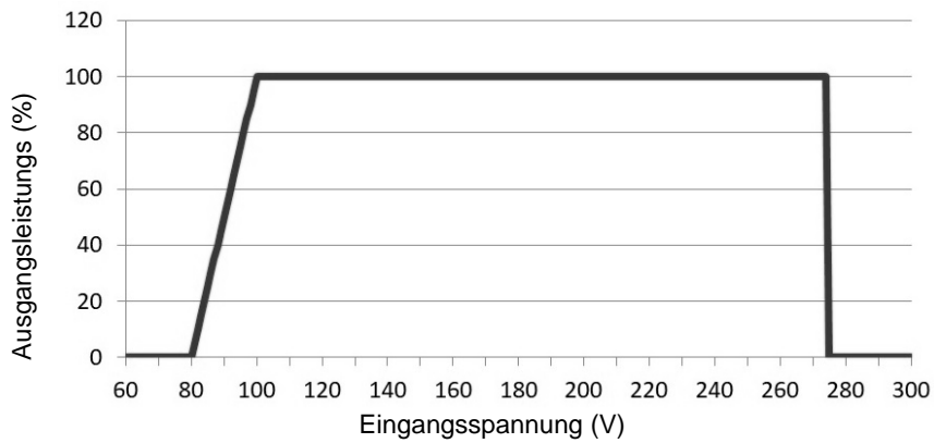
Abbildung 8: Ausgangsleistung zur Eingangsspannung
