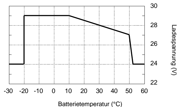
Abbildung 7: Laden mit Temperatenausgleich
