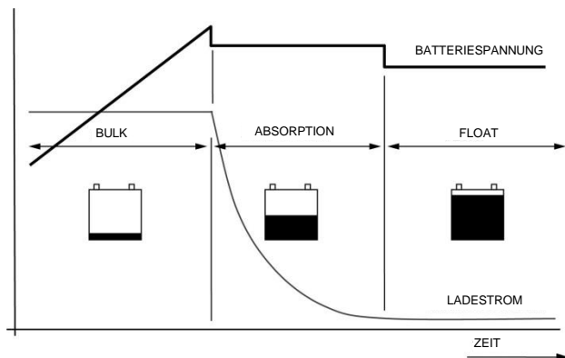
Abbildung 6: 3-stufiger Ladevorgang
