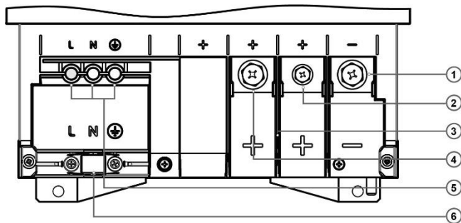
Vorderseite mit offenem Anschlussbereich
