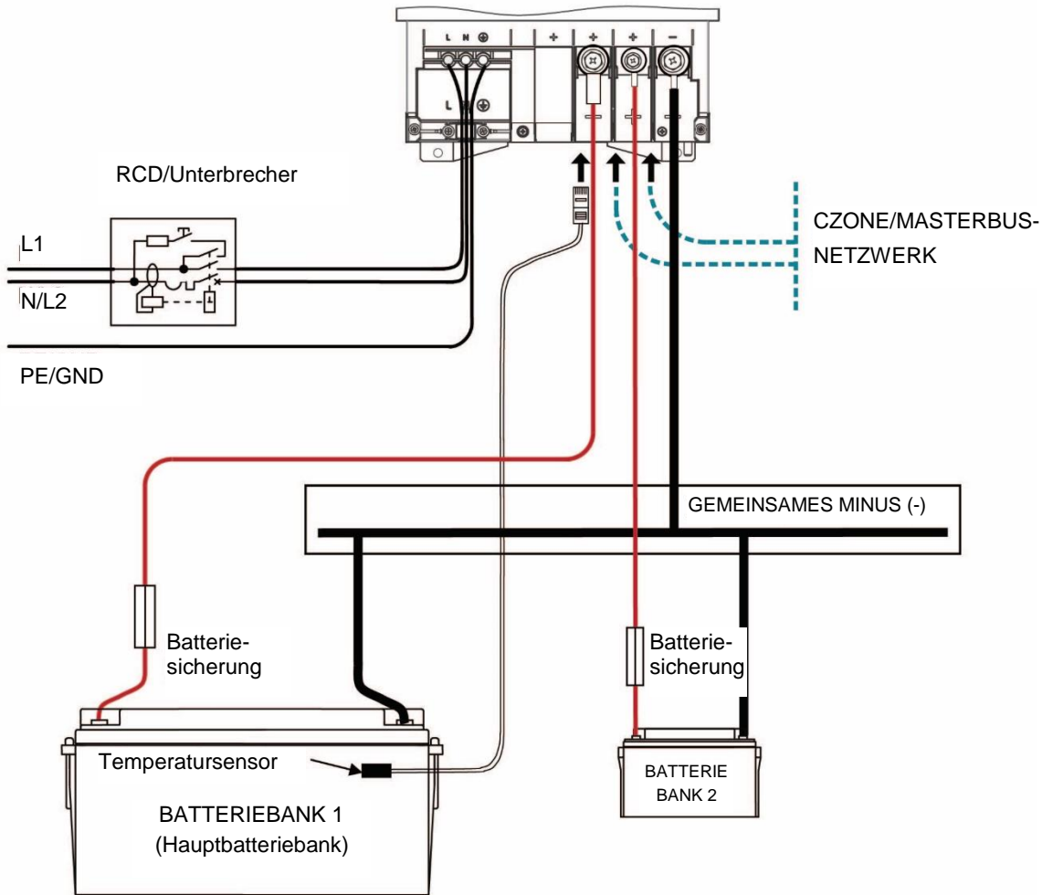
Abbildung 3: Installationsschema des ChargeMaster Plus
